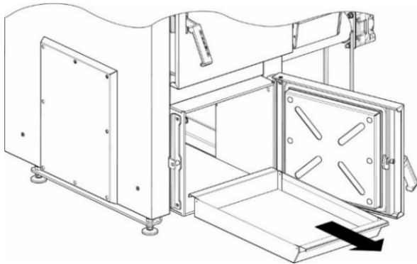
Rysunek 15. Sposób usuwania popiołu z kotła.
