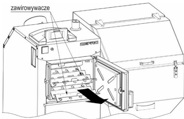
Rysunek 14. Sposób demontażu zawirowywaczy.
