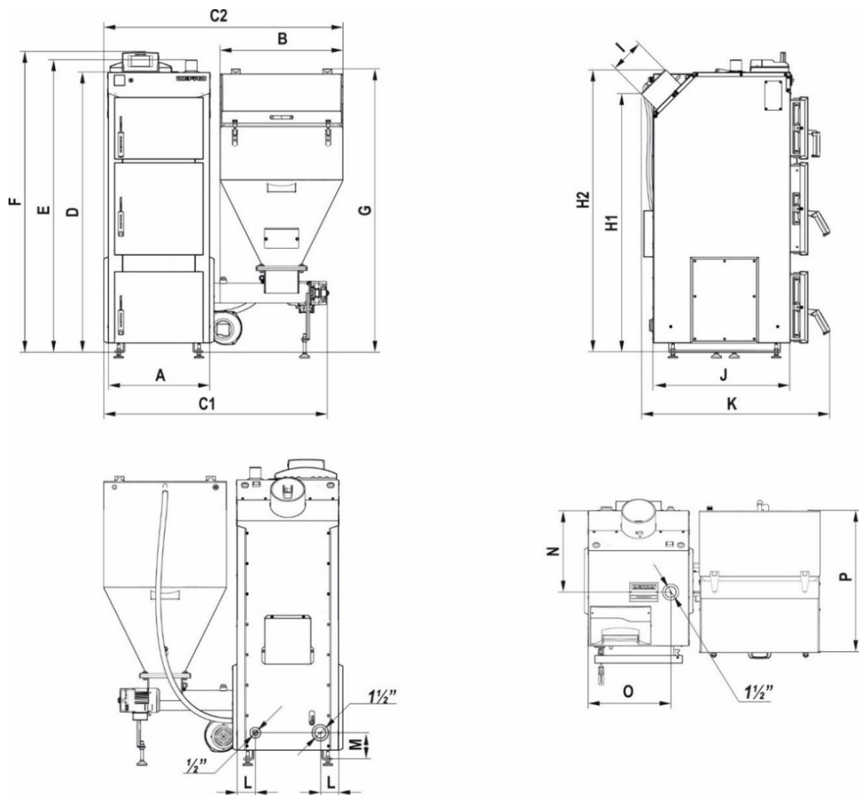
Rysunek 2. Podstawowe wymiary kotła KOMFORT EKO LUX.
