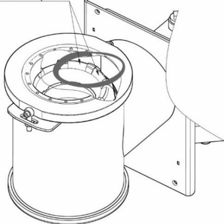
KROK 5. Zmontować palnik retortowy zwracając uwagę, aby przesłony znajdowały się na wprost rury podawczej podajnika.
